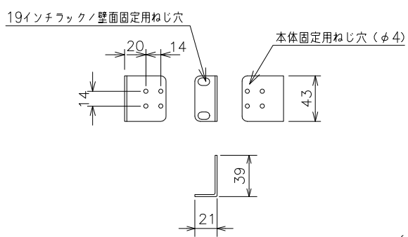
19インチラック固定用金具 (同梱)
